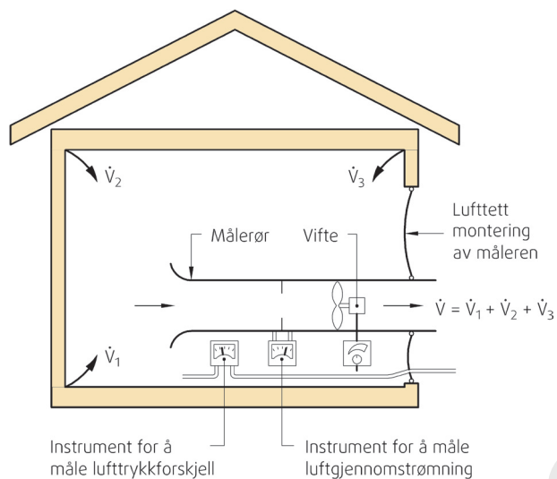
Fig. 21 Trykkmetoden, måleprinsipp
